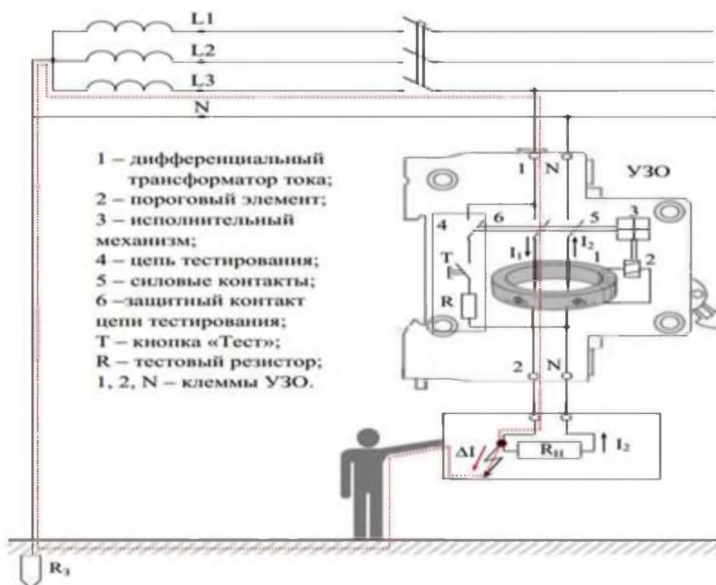
Рисунок 3. Принцип работы УДТ
