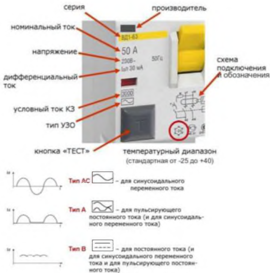
Рисунок 5. Маркировка УДТ
