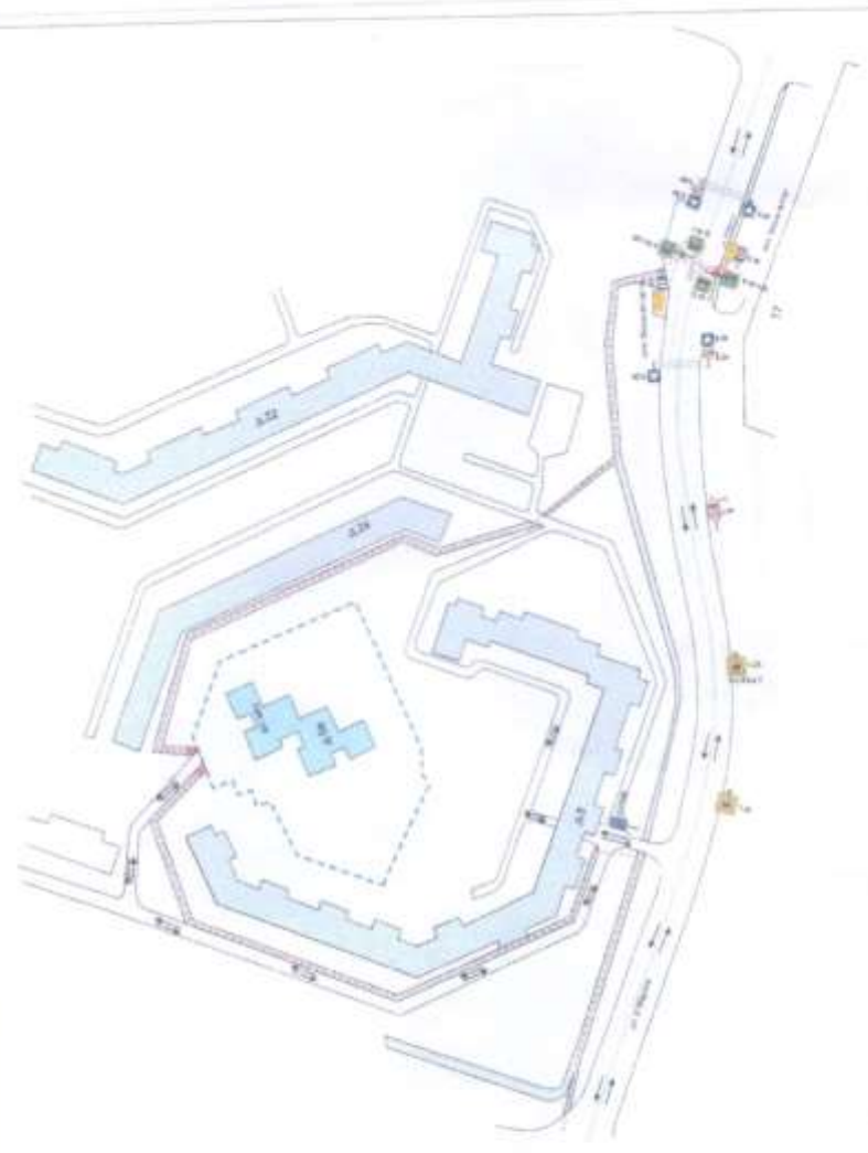
План-схема образовательного учреждения и организации дорожного движения в непосредственной близости от образовательного учреждения с размещением соответствующих технических средств организации дорожного движения детей (обучающихся, воспитанников), транспортных средств
