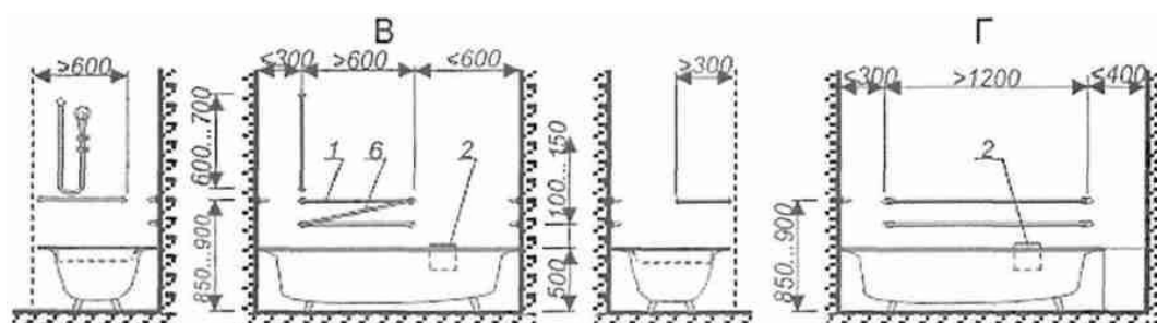
Варианты планировки ванной комнаты
