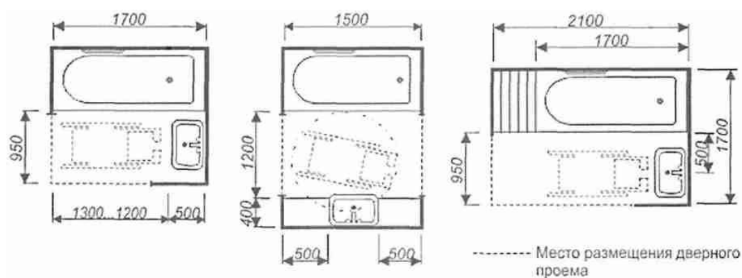
Варианты планировки ванной комнаты
