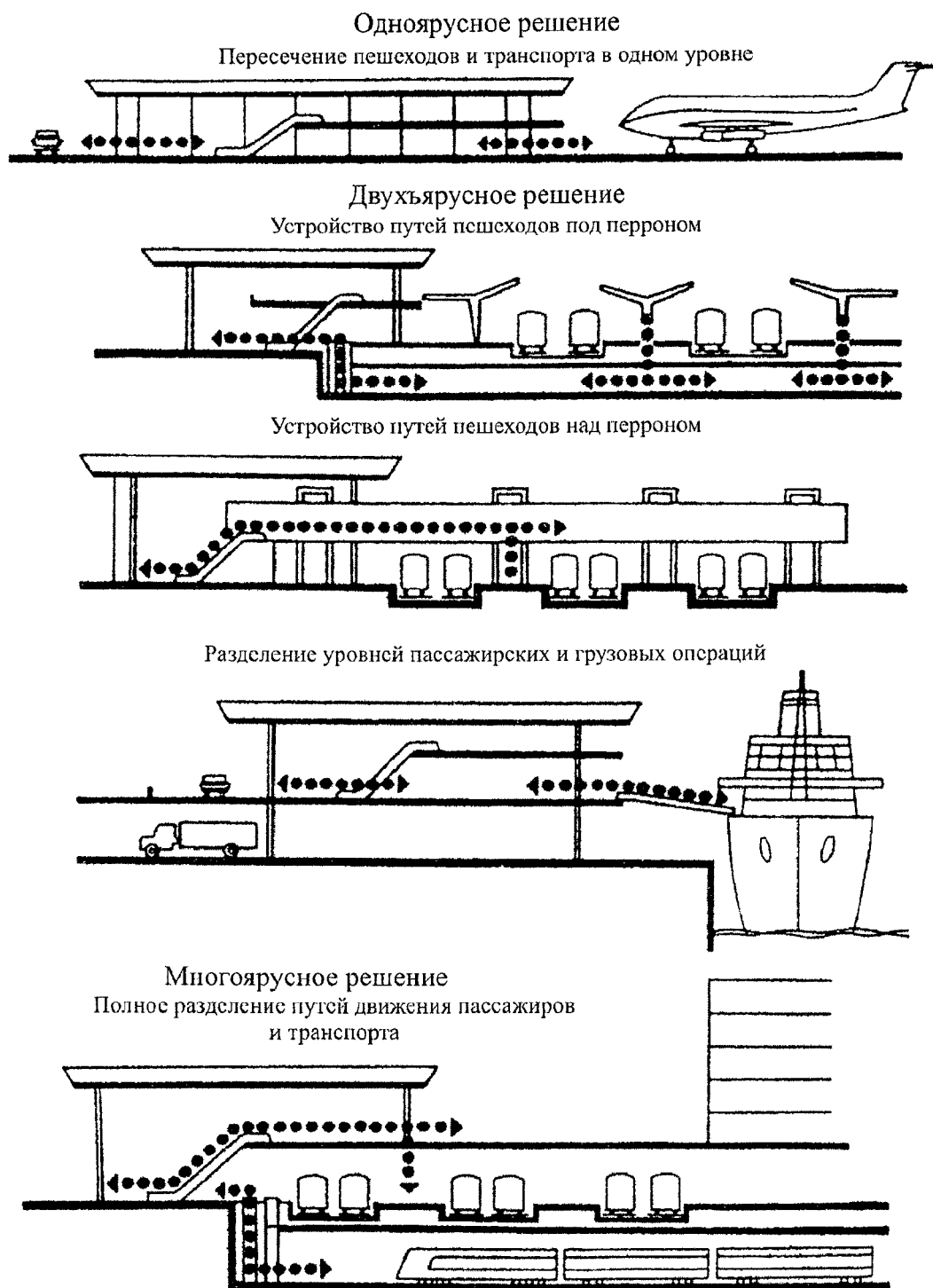
Рисунок В.8. Приемы организации движения пассажиров в вокзальных комплексах различного назначения
